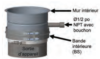
Schéma 77 - Adaptateur simple paroi avec port d'essai (SWAN) installé sur un appareil
