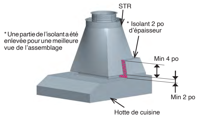
Schéma 100: Transition du STR - hotte de cuisine à un conduit de graine
