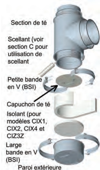
Schéma 33a: Capuchon de té étape 1
