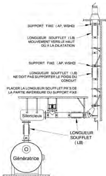
Schéma 53- Localisation des longueurs soufflet
