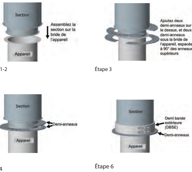
Schéma 80 - Installation de l'adaptateur demi-anneau universel (HUF) sur un appareil avec une bride de 1/2 po (aucun trous)
