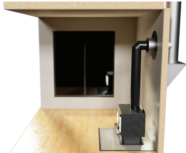
INSTALLATION TRAVERSANT UN MUR
