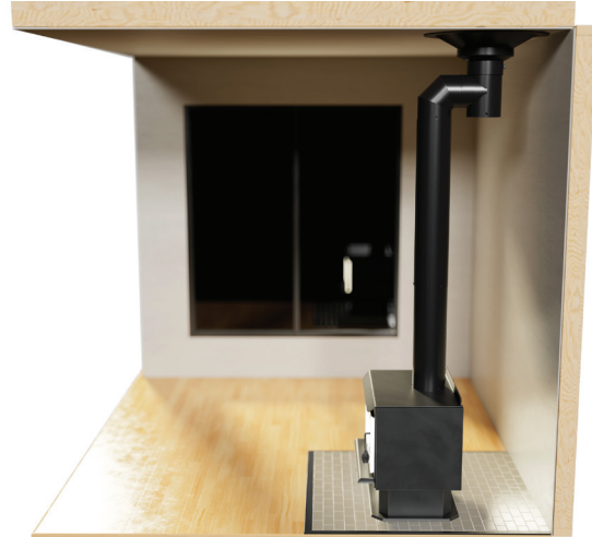
INSTALLATION AVEC TÉ DE NETTOYAGE
