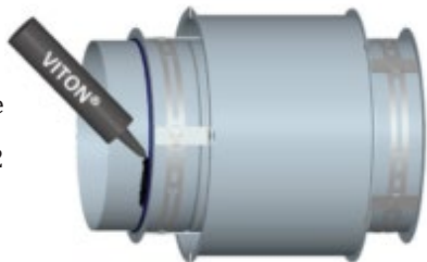
Assemblage de Section Étape 2
