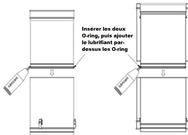
Figure 11 - Longueur télescopique
