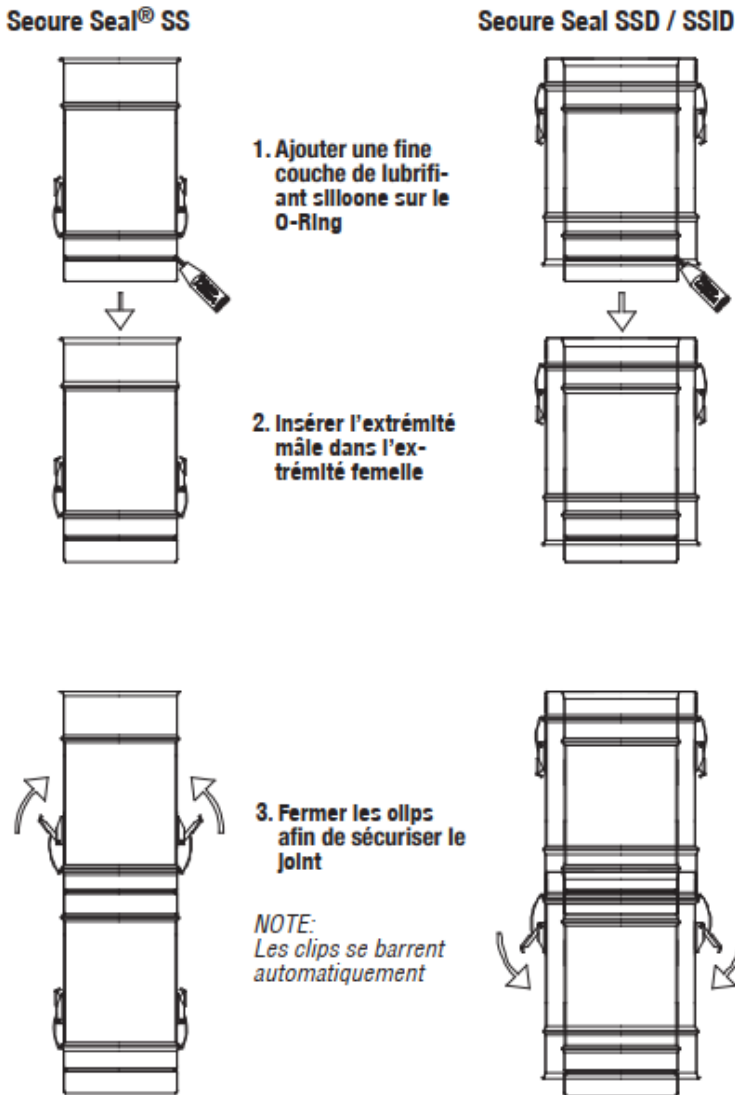
Figure 7 - Étapes d'assemblage de sections
