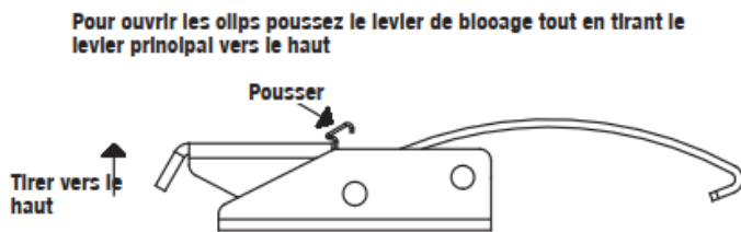
Figure 8 - Pour ouvrir le Loquet
