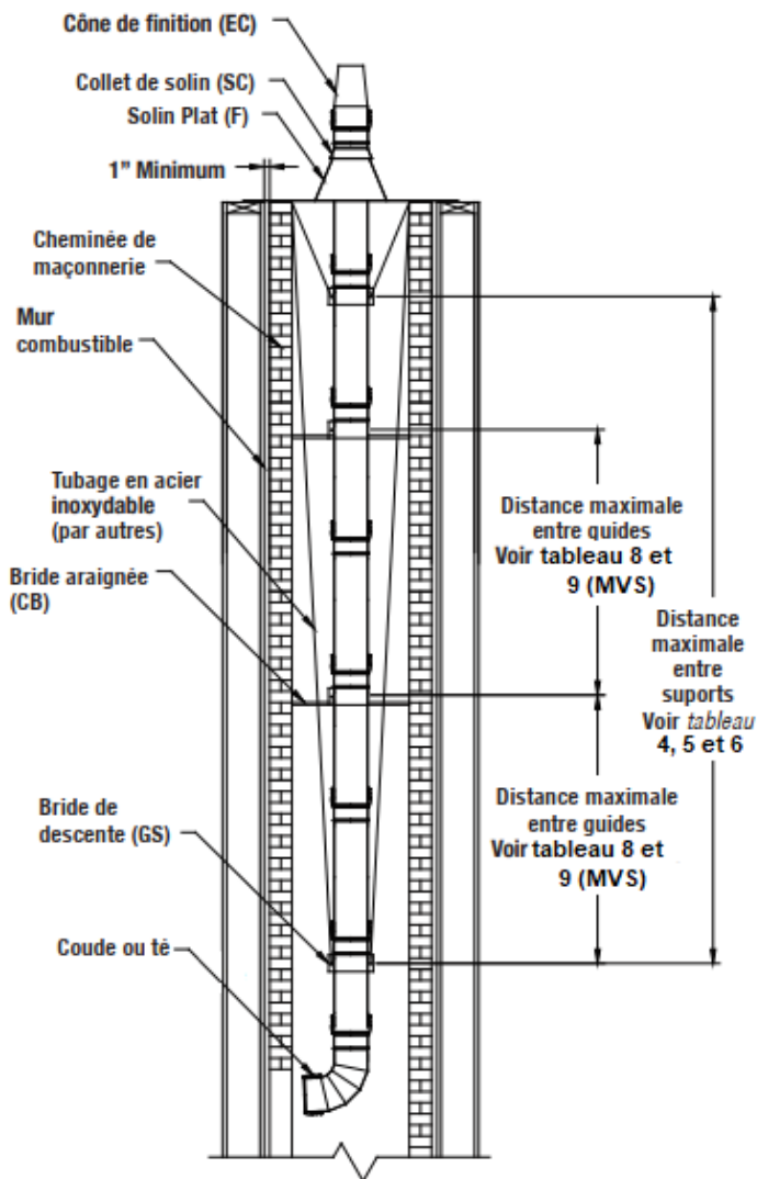
Figure 12 - Installation de Secure Seal comme tubage
