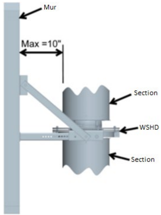
Figure 54c: Réglage maximal WSHD
