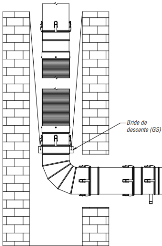
Figure 25 - Adaptateur Secure Seal Flex - Coude en maçonnerie
