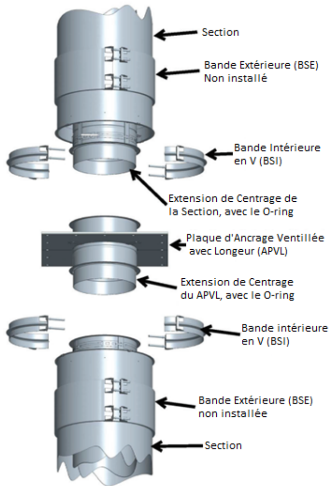
Figure 51: Étape 1 de l'installation d'APVL
