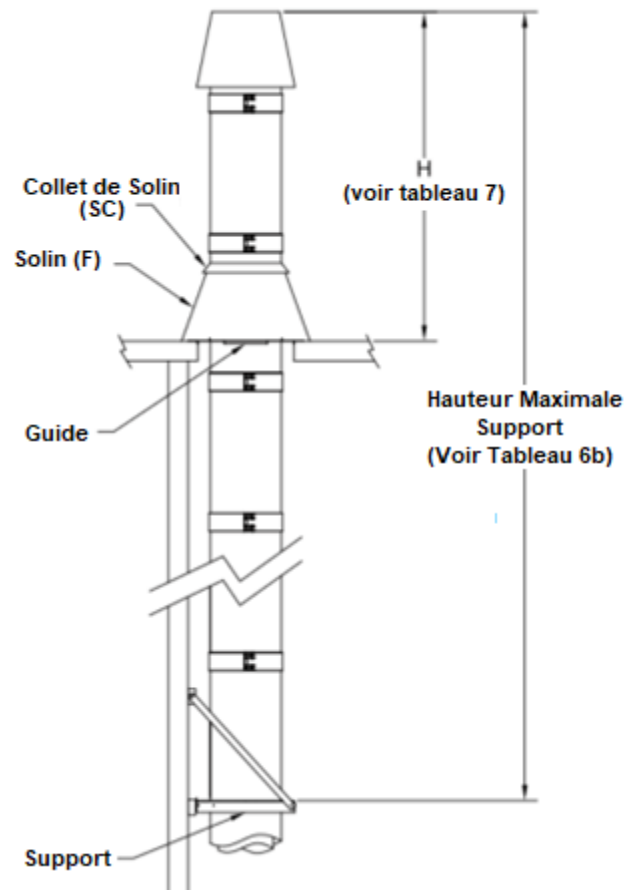
Figure 28 - Hauteur autoportante maximale pour les LDCS
