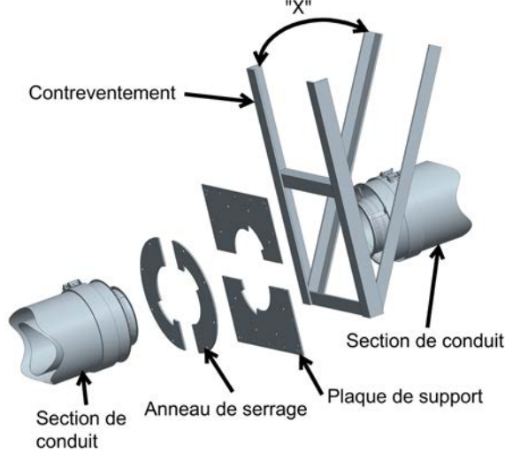
Schéma 42 - Plaque d'ancrage sur contreventement
