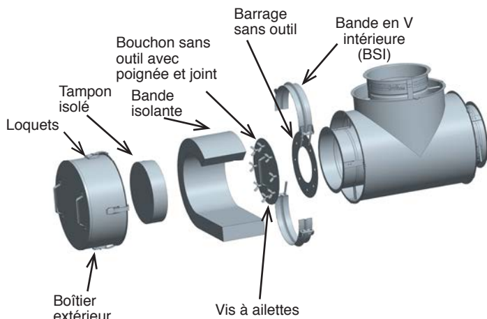
Schéma 90- Bouchon de té sans outil (NTTC)
