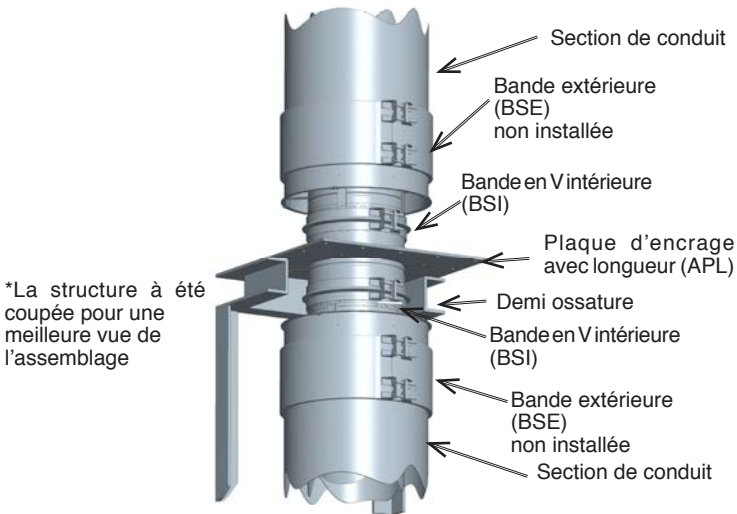
Schéma 45 - Étape 2 de l'installation de l'APL
