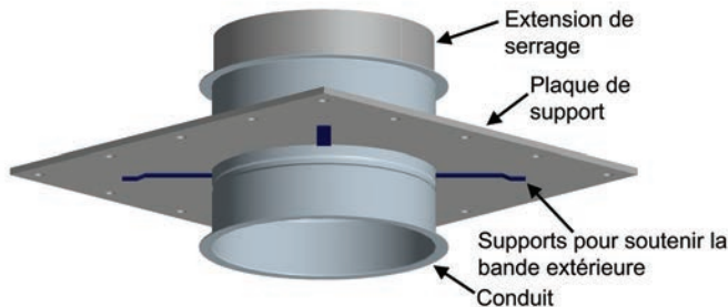
Schéma 43 - Plaque d'ancrage avec longueur (APL)
