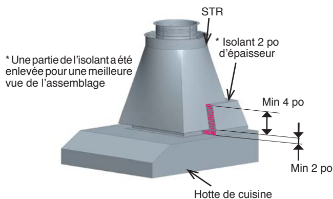
Schéma 100: Transition du STR - hotte de cuisine à un conduit de graisse
