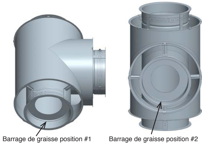
Schéma 93a - Barrage de graisse position #1
