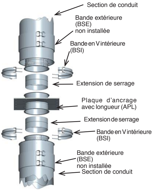
Schéma 44 - Étape 1 de l'installation de l'APL
